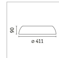
Jaron Ceiling luminaire 96784 □ p. 54
