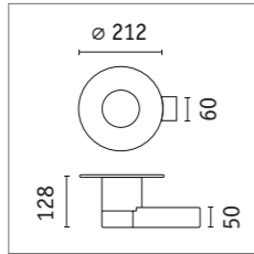
Sienna Wall luminaire IP44 94834 □ p. 57
