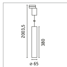
ProRail3 pendant 95398 □ p. 52
