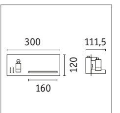
Serra Wall luminaire 71102 □ p. 55
