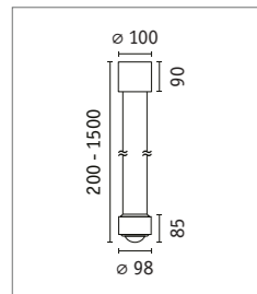
Aldan URail pendant 95520 □ p. 52
