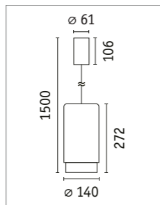
Corus URail Pendant 95401 □ p. 53
