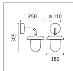
Vintario Wall luminaire IP44 94757 □ p. 57
