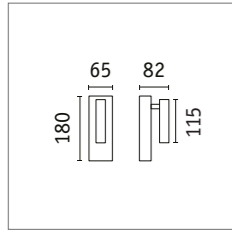
Hulda Wall luminaire 71108 □ p. 55
