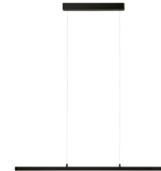
Lento Pendant luminaire incl. 1x42 W 1.800 lm, 2.700 K 230 V ⌀25 mm ⌀6,7-150 cm ⌀1.000 mm ⌀35 mm 79693
