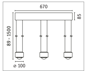
Aldan Pendant luminaire 79720 □ p. 55
