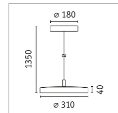
Hildor Pendant luminaire 96782 □ p. 55
