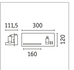
Serra Wall luminaire 71103 □ p. 55
