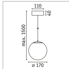
Gove Pendant luminaire IP44 71066 □ p. 51
